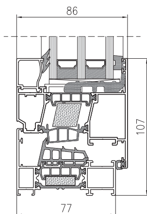
PRŮŘEZ OKNA TM 62HI OUTWARD
