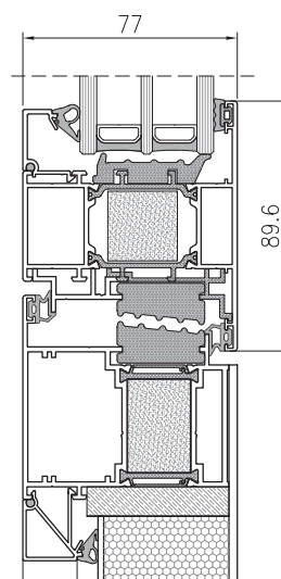
TM 77HI PRESTIGE AJTÓN ÁTMENŐ METSZET
