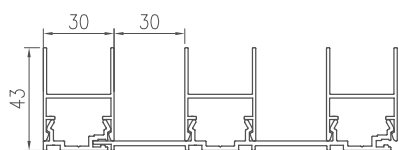
PRZEKRÓJ PRZEZ OKŁADZINE ŚCIENNĄ VERTILINE
