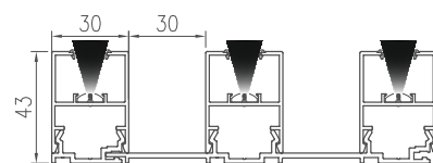
PRZEKRÓJ PRZEZ OKŁADZINE ŚCIENNĄ VERTILINE - LED
