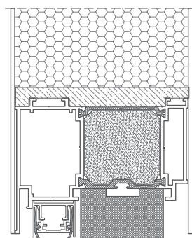
PRZEKRÓJ ROZWIĄZANIA TM 77HI
