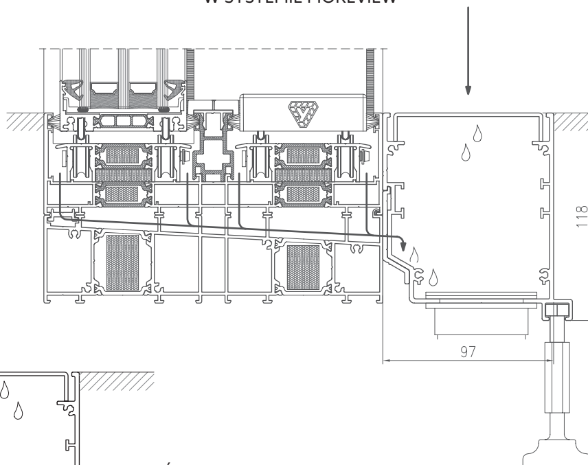
PRZEKRÓJ ROZWIĄZANIA TM 77HI
