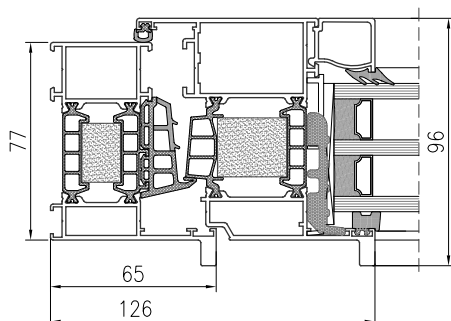
PRZEKRÓJ PRZEZ OKNO TM 77HI INDUSTRIAL
