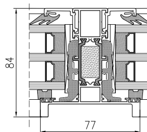
PRZEKRÓJ PRZEZ SŁUPEK TM 74HI INDUSTRIAL
