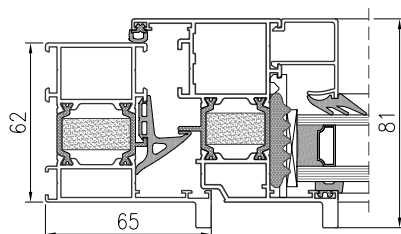
PRZEKRÓJ PRZEZ OKNO TM 62HI INDUSTRIAL
