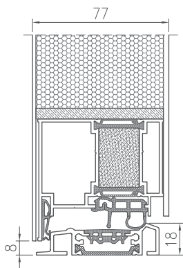
PRZEKRÓJ PRZEZ DRZWI TM 77HI PRESTIGE
