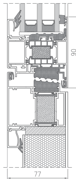
PRZEKRÓJ DRZWI TM 77HI PRESTIGE Z NAŚWIECIEŁEM
