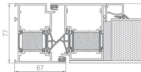
PRZEKRÓJ PRZEZ DRZWI TM 77HI PRESTIGE
