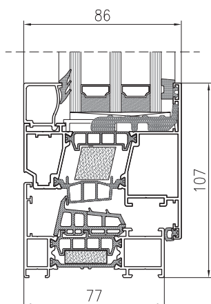
PRZEKRÓJ PRZEZ OKNO TM 77HI OUTWARD
