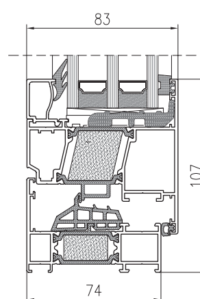
PRZEKRÓJ PRZEZ OKNO TM 74HI OUTWARD
