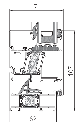
PRZEKRÓJ PRZEZ OKNO TM 62HI OUTWARD
