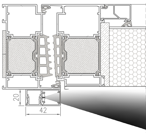
PRZEKRÓJ PRZEZ DRZWI Z PROFILEM DO MONTAŻU OŚWIETLENIA LED
