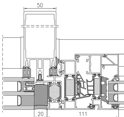
PRIEREZ STĹPOM FA 50N SL S OKNOM TM 77N
